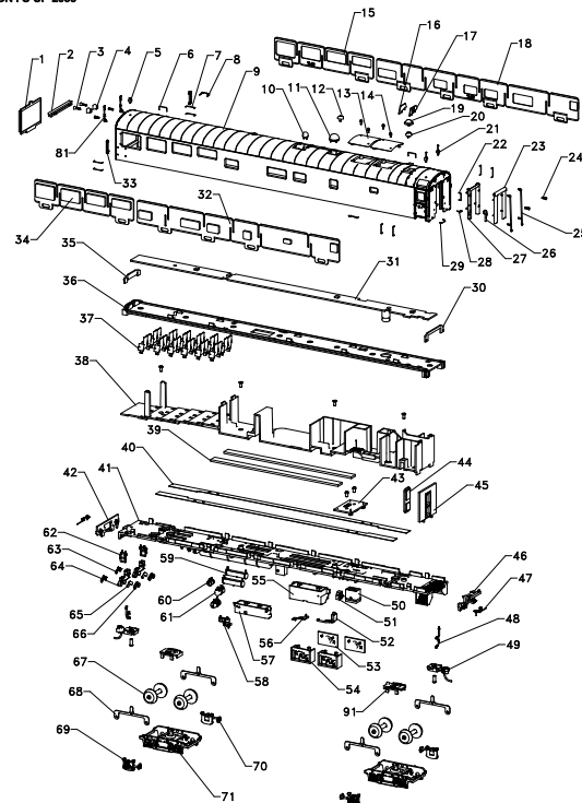
BCH02-EXPLODE VERSION : C-UP-2006
