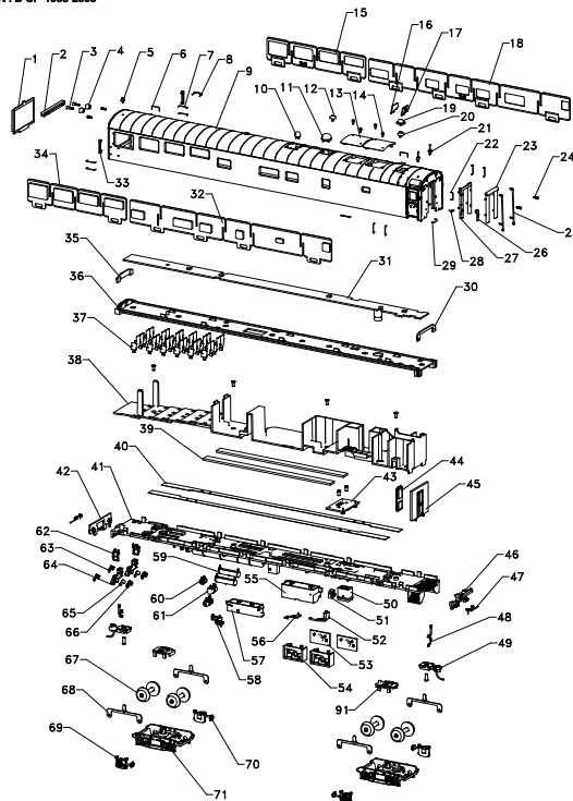
BCH02-EXPLODE VERSION : B-UP-1995-2006
