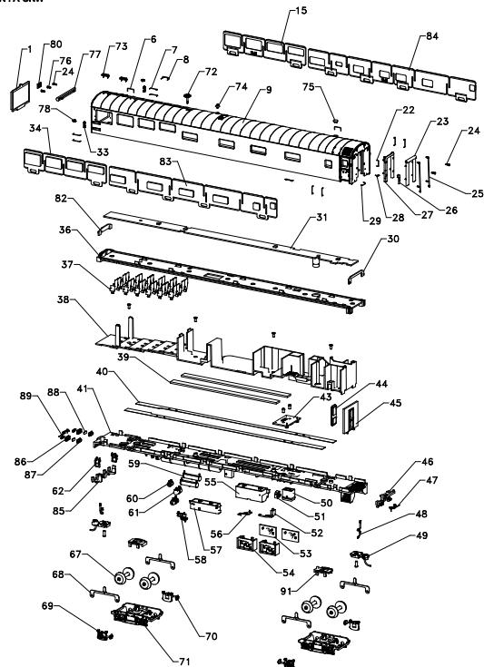
BCH02-EXPLODE VERSION : A-CNW
